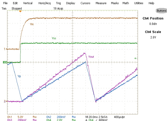
Fig. 7: Start up at 7A Load, V_p: 0.6V Ch 1 : V_{in} , Ch 2 : V_{SS} , Ch 3 : V_{out} , Ch 4 : I_{out}
