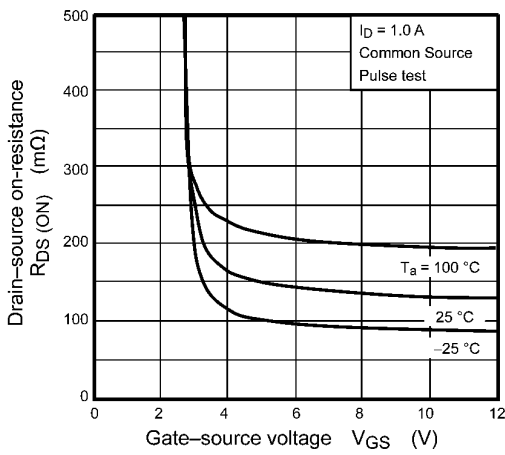
Fig. 7.3 R_{DS(ON)} - V_{GS}
