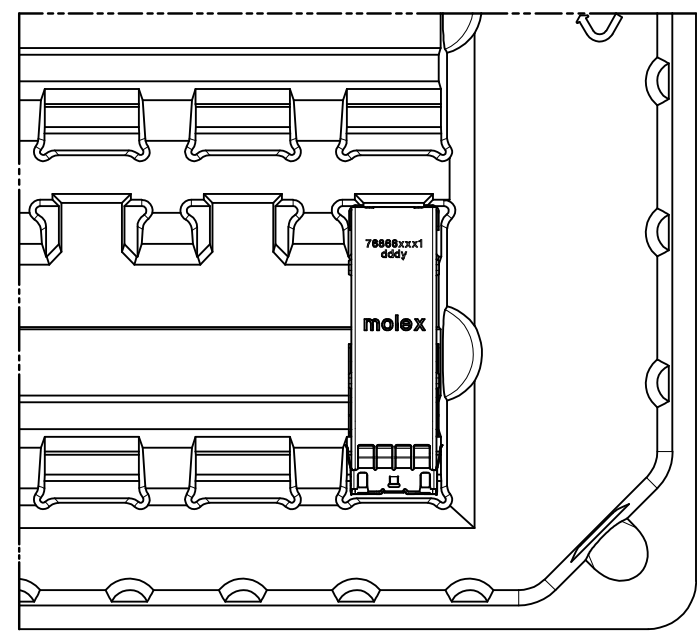
Partial1 SCALE 1:1
