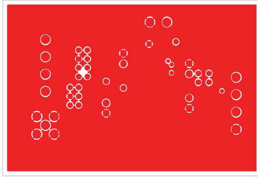
Figure 11. EVAL-ADM3065EEBZ/EVAL-ADM3065EEB1Z Layer 4
