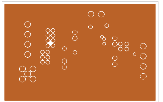
Figure 9. EVAL-ADM3065EEBZ/EVAL-ADM3065EEB1Z Layer 2
